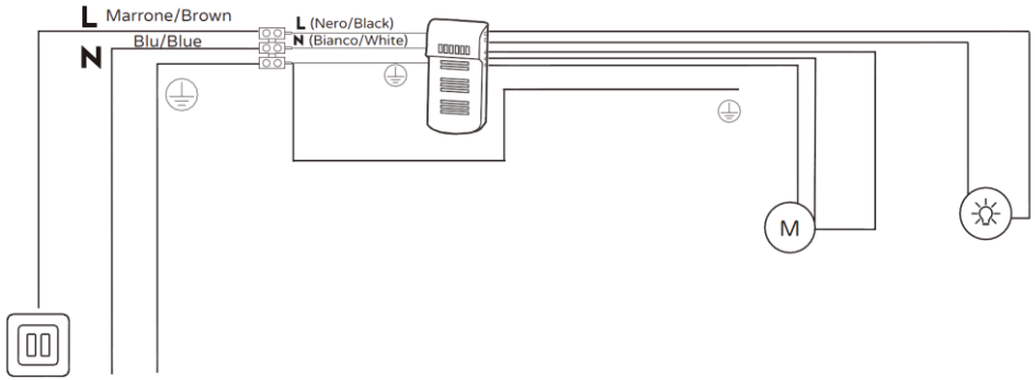
Interruttore a parete/ Wall controls
